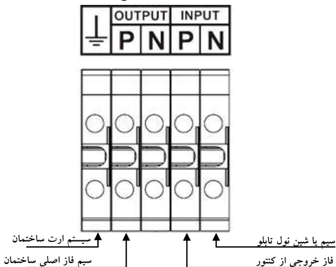
شکل 3. ترمینال‌های ورودی و خروجی دستگاه
