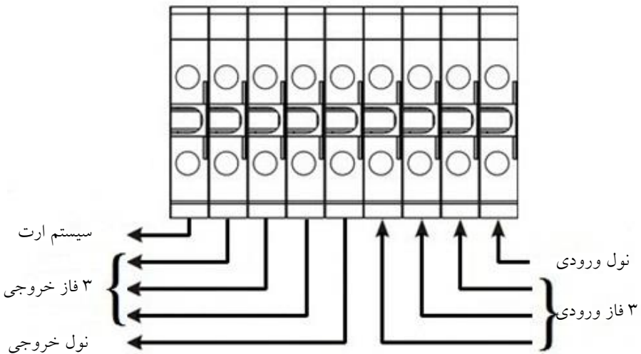
شکل ۲- ترمینال های ورودی و خروجی دستگاه
